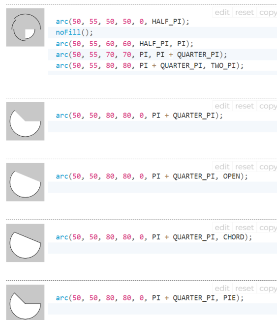
Figura 1.2. Exemple de desenare a arcurilor
