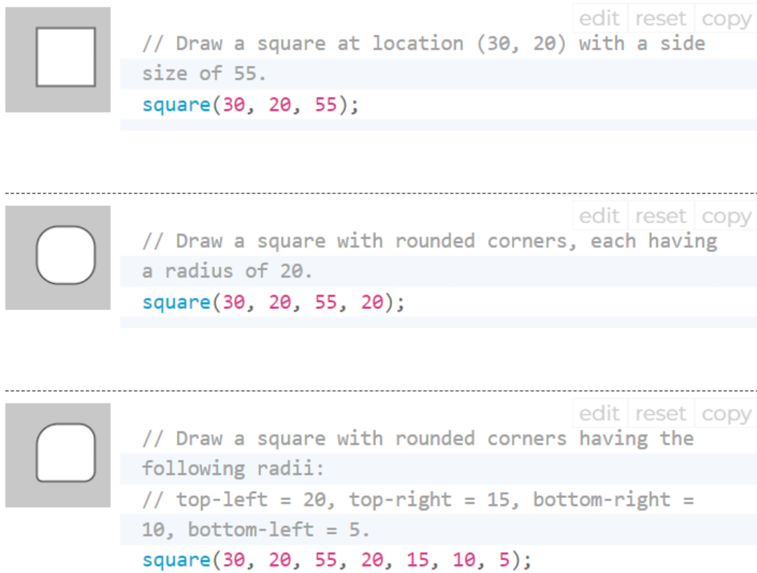
Figura 1.7. Exemplu de utilizare a funcției square
