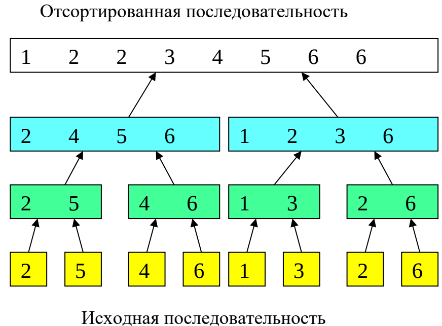
Рисунок 2.1 - Сортировка слиянием для массива A [5, 2, 4, 6, 1, 3, 2, 6]
