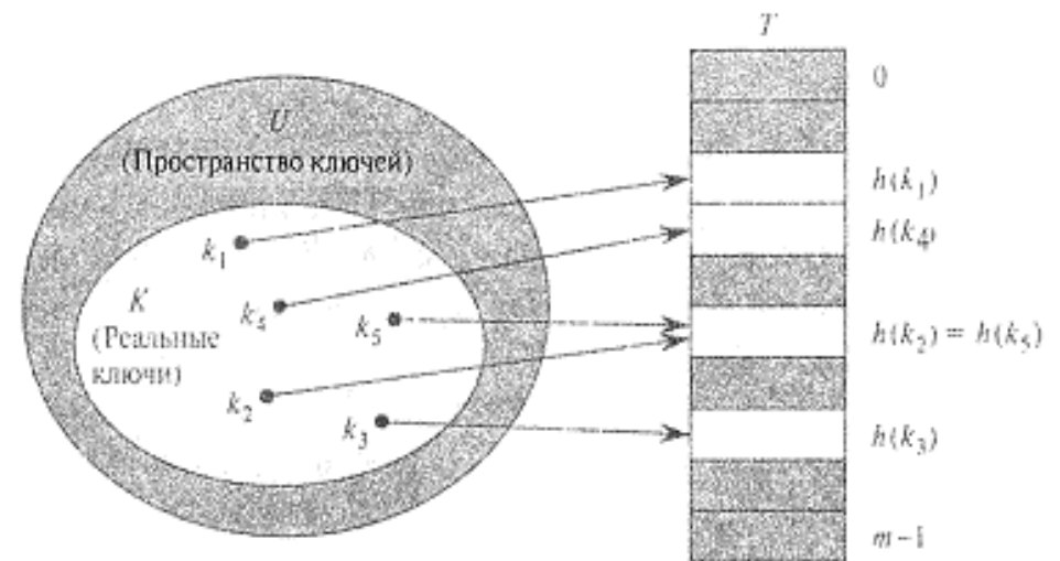
Рисунок 9.2 – Использование хеш-функции для отображения ключей в позиции хеш-таблицы. Хеш-значения ключей k_2 и k_5 совпадают- имеет место коллизия
