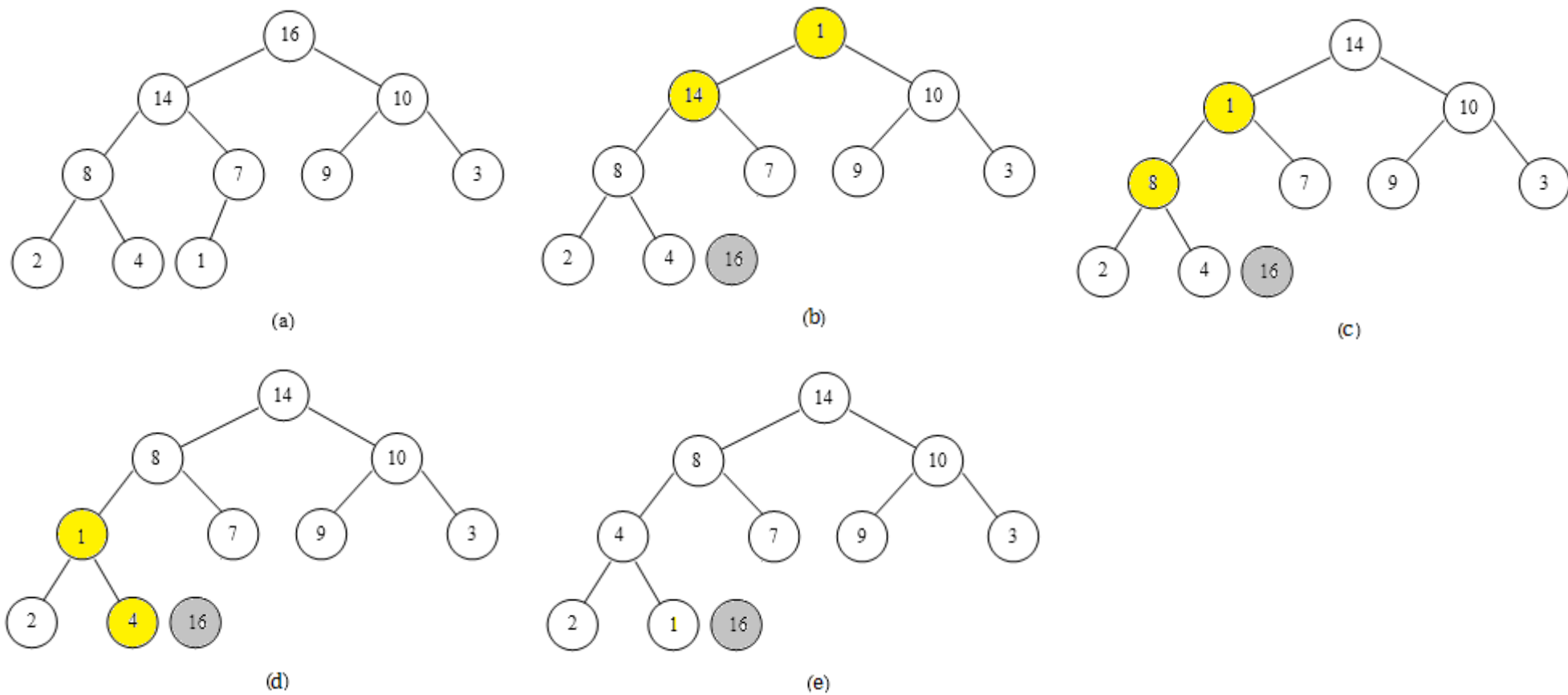
Рисунок 5.5 – Демонстрацию работы процедуры HEAPIFY(A,1)
