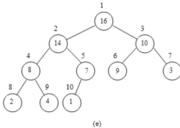
Рисунок 5.3 - Работа процедуры BUILD-HEAP. Показано состояние данных перед каждым вызовом процедуры HEAPIFY в строке 3
