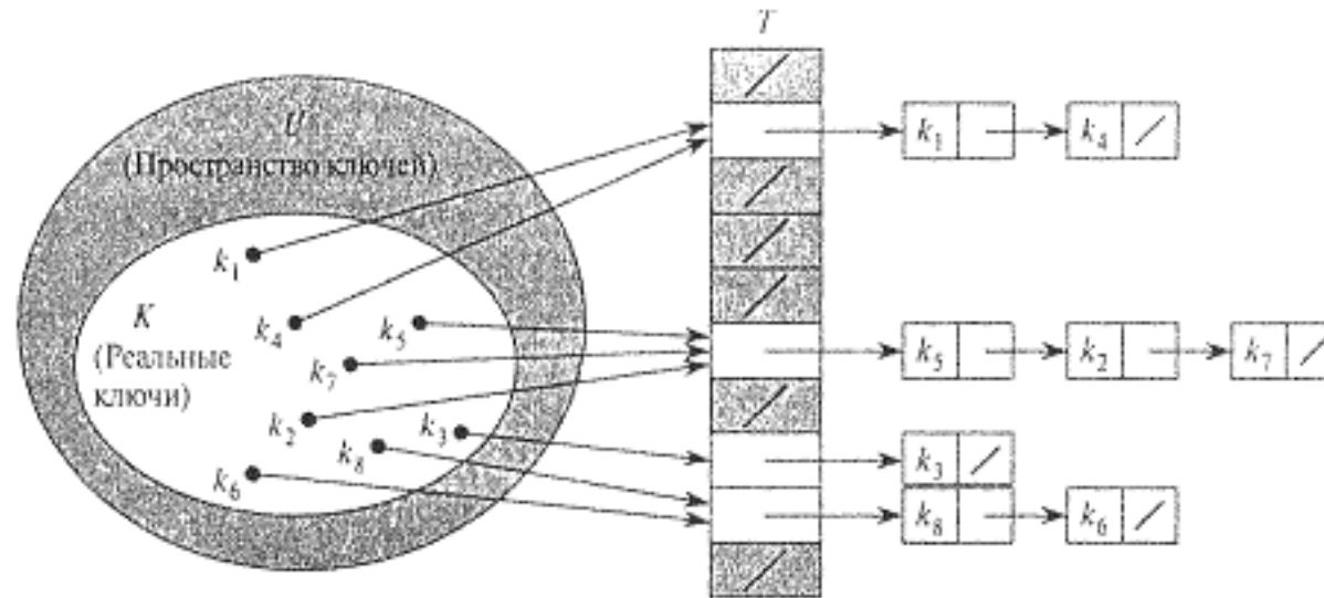
Рисунок 9.3 – Разрешение коллизии с помощью цепочек. В позиции T[j] хранится указатель на список элементов с хеш-значением j . Например, h(k_1) = h(k_4) и h(k_5) = h(k_2) = h(k_7)
