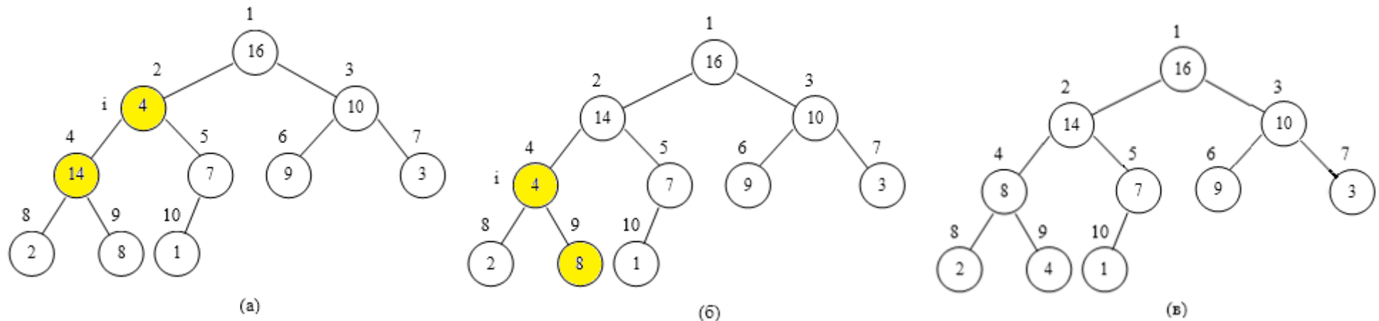
Рисунок 3.2 - Работа процедуры \text{HEAPIFY}(A, 2) при \text{heap-size}[A] = 10 .
