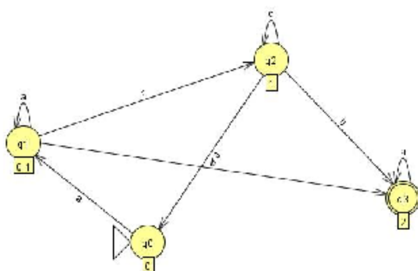
Граф ДКА (под узлами графа подписаны индексы состояний из графа НКА)
