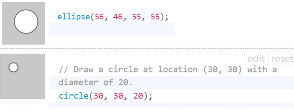
Figura 1.4. Exemple de program și rezultatul acestuia pentru funcțiile circle și ellipse
